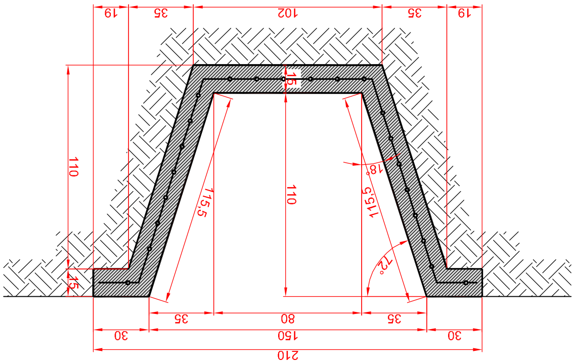
SECȚIUNE TRANSVERSALA TIP
